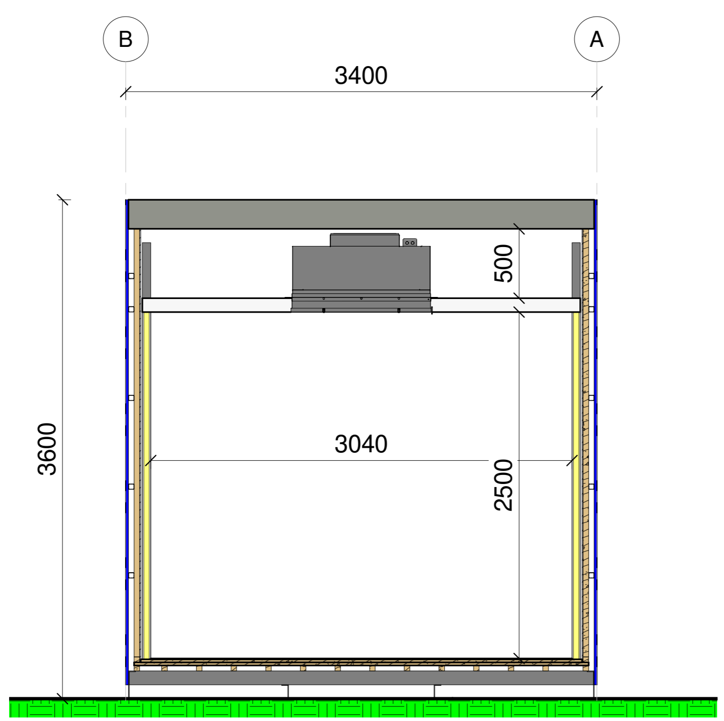
5 Section 1 1:25
