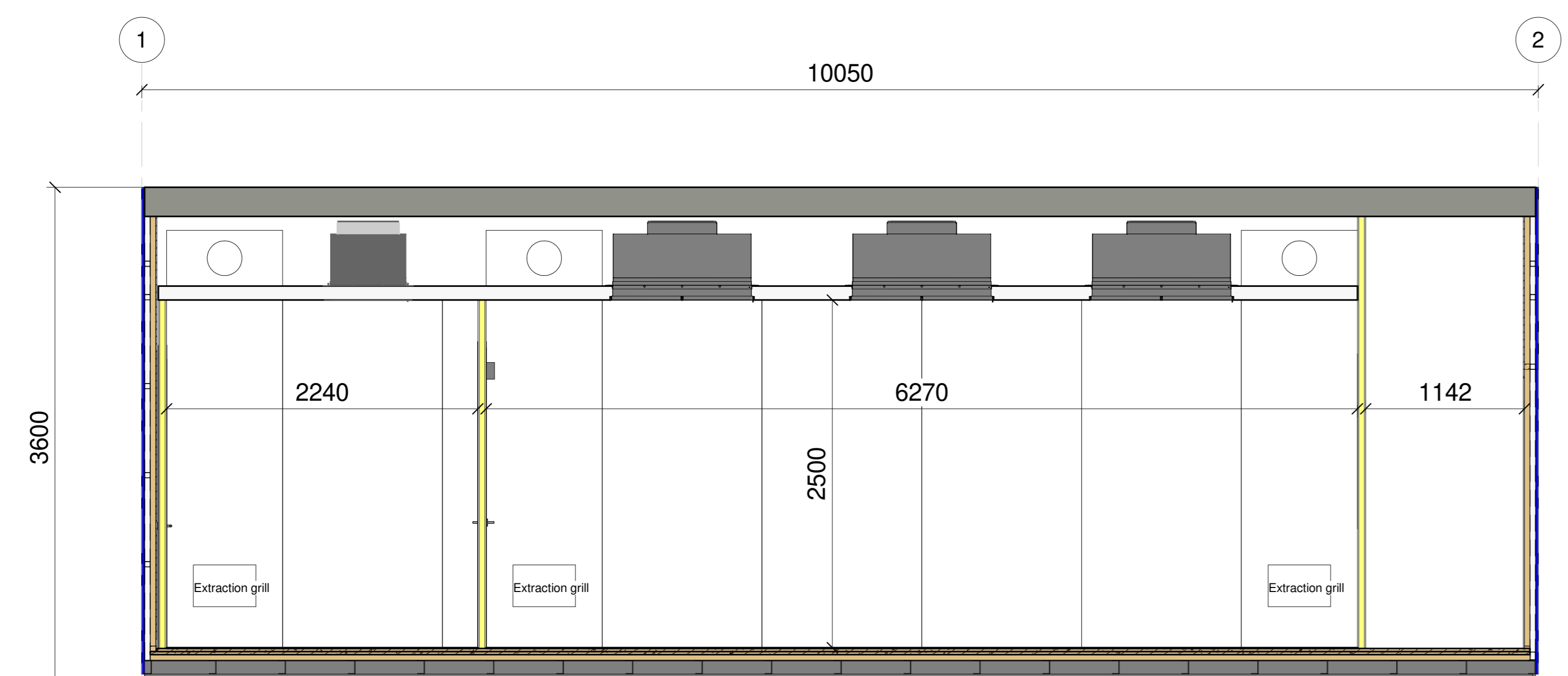
6 Section A 1:25
